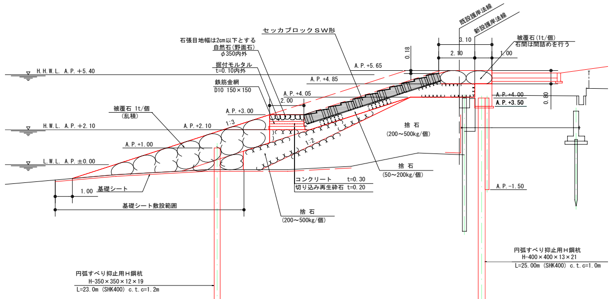
標準断面図
